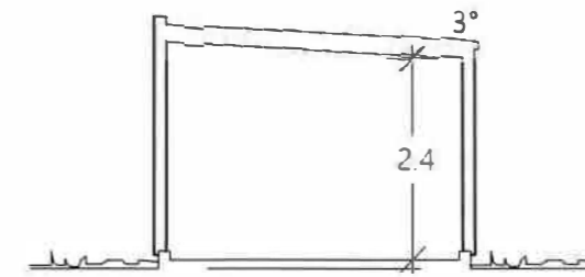
SEKTION A-A
